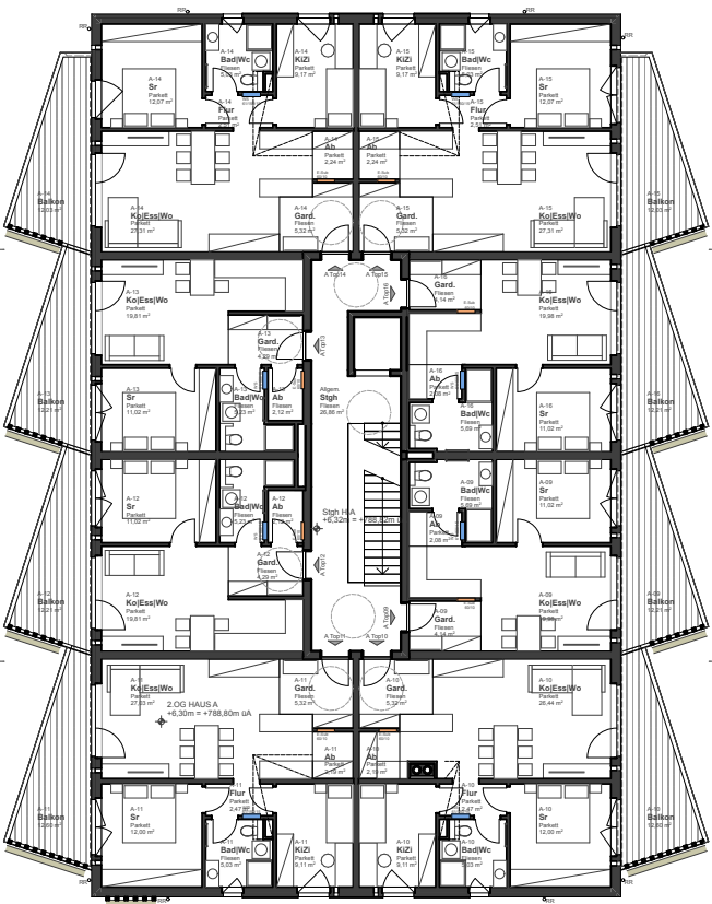
2. OBERGESCHOSS
