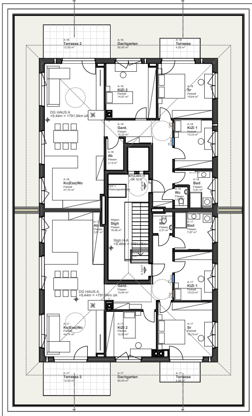
DACHGESCHOSS
